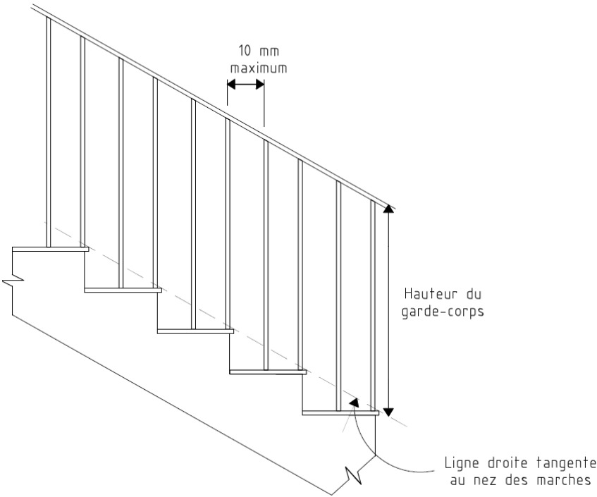
Dimensionnement d'un garde-corps
