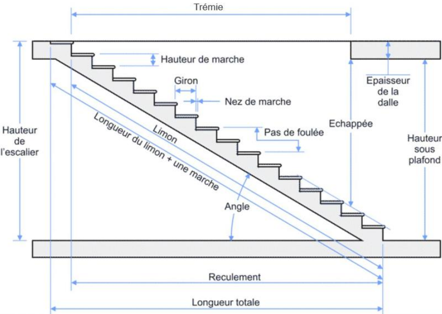
Les éléments constitutifs d'un escalier
